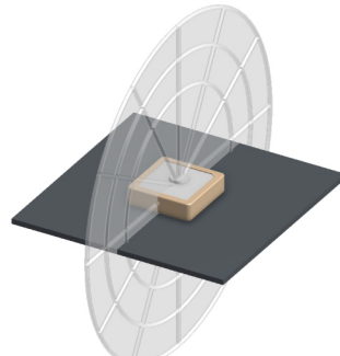
YZ-Plane Gain
