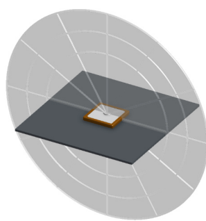
XZ-Plane Gain
