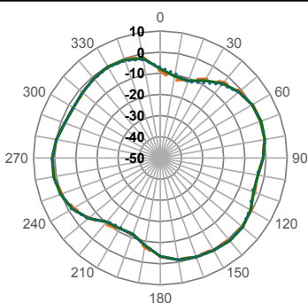
XZ-Plane Gain
