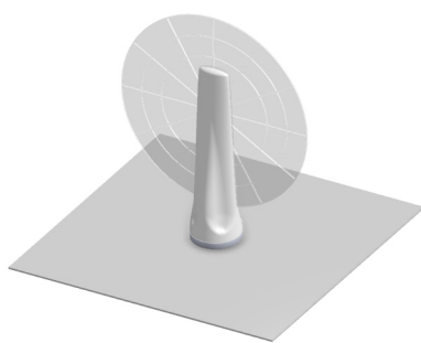
XZ-Plane Gain
